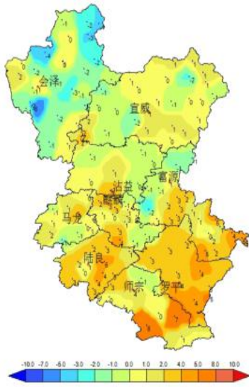
图1 2023年1月1日08时至1月6日08时最低气温（单位：℃）
